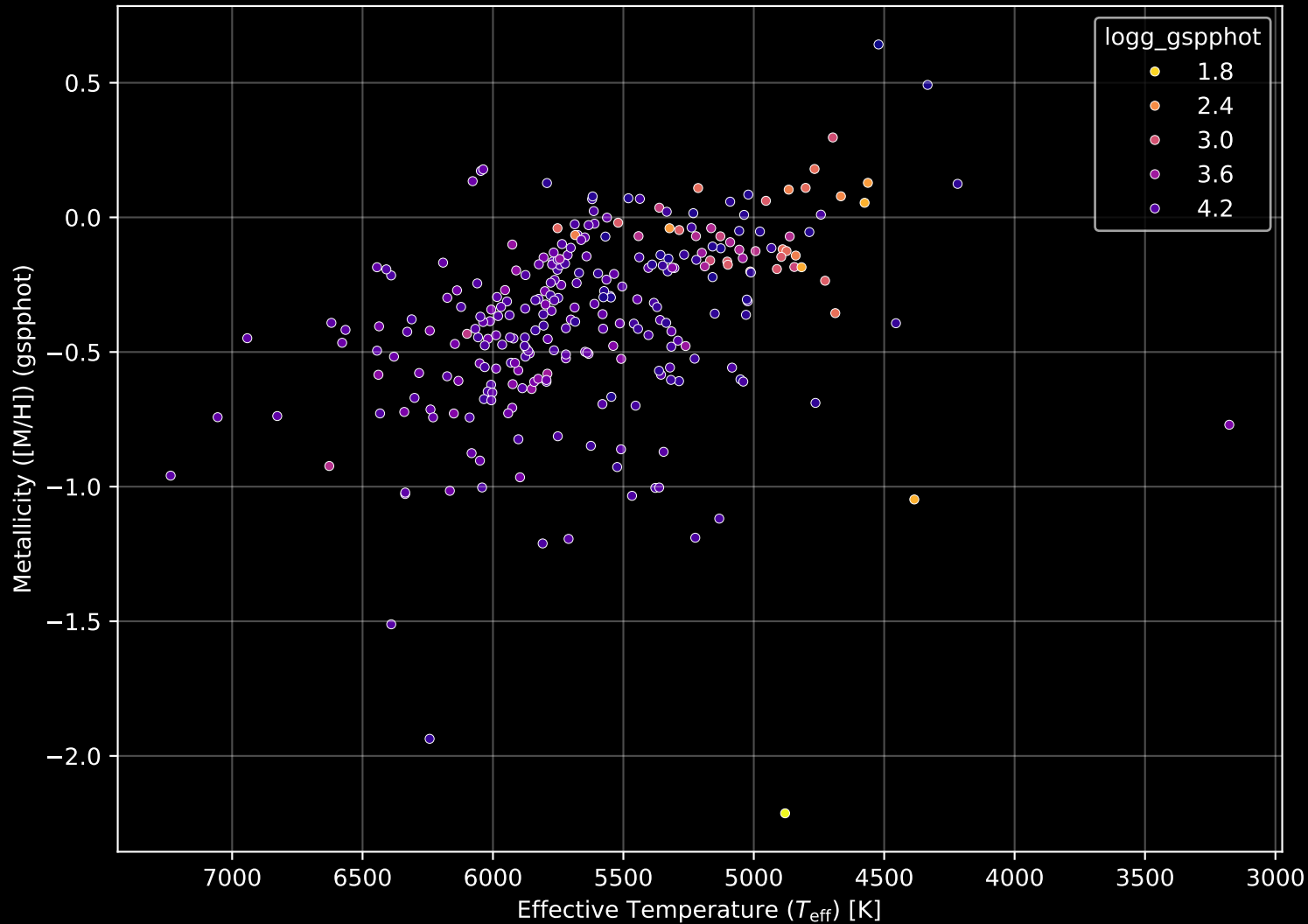
GALAH DR4 Field: [446] Stellar Population Parameters (n= 279)
