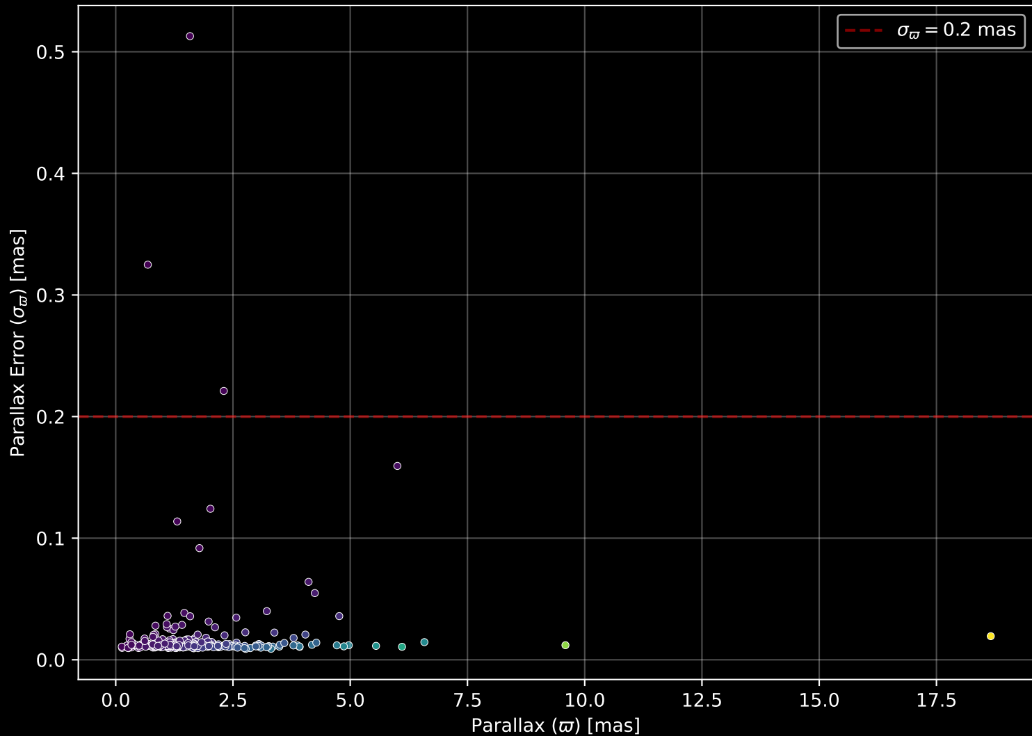
GALAH DR4 Field: [446] Parallax Quality (n= 279)
