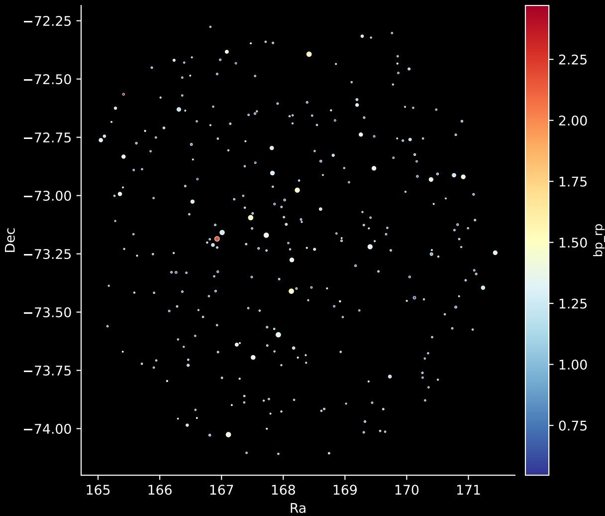
GALAH DR4 Field: [446] Stars: 279
