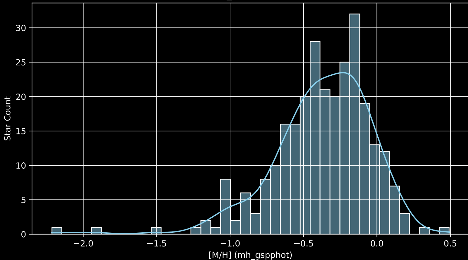
GALAH DR4 Field: [446] [M/H] (mh_gspphot) (n= 278)
